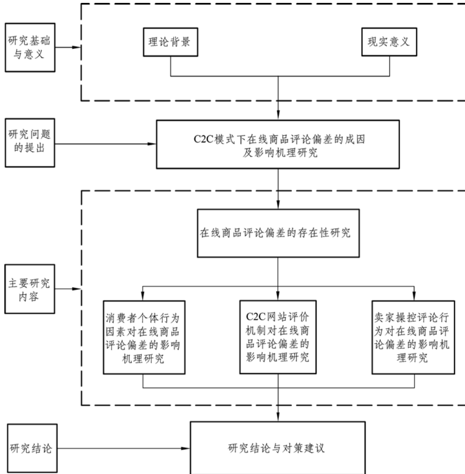
图 1.4 逻辑框架
