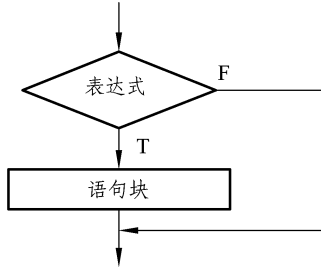
图 1.2 单分支结构
