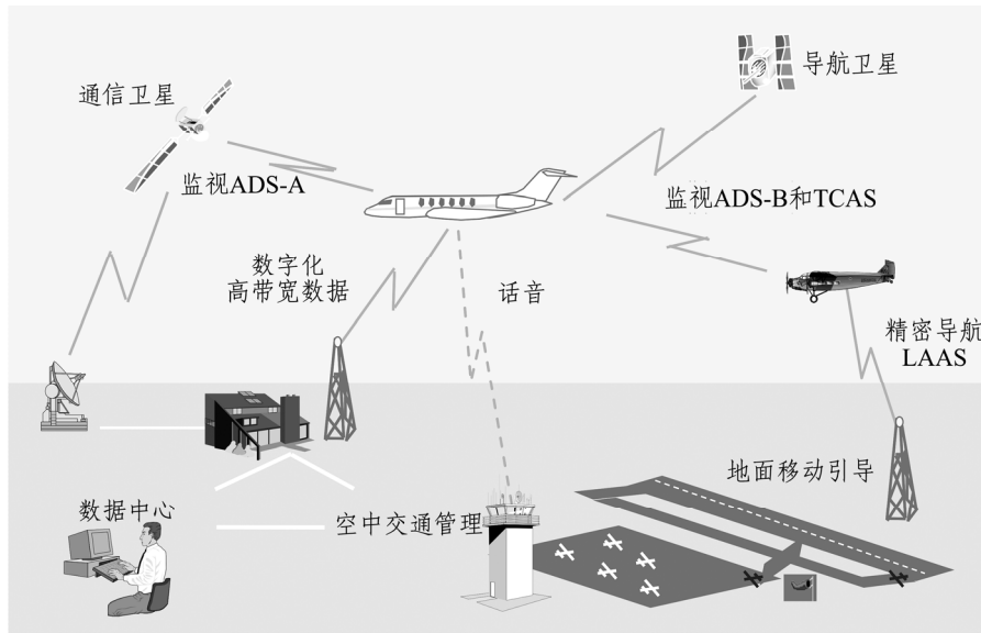
图 1.1 CNS/ATM 环境
