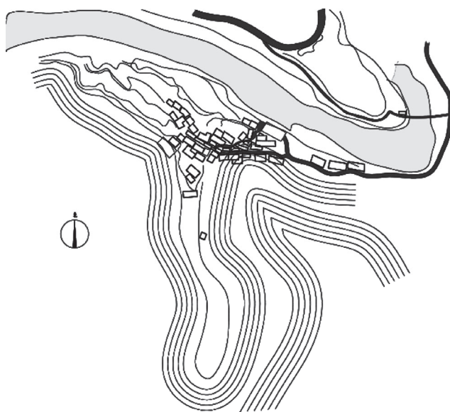
图 2-4 季刀上寨总平面图
