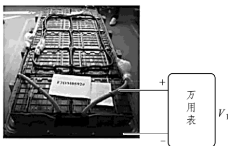
图 1-27 选择 V_{\text{正}} 和 V_{\text{负}} 中较大的值重测并记为 V_1
