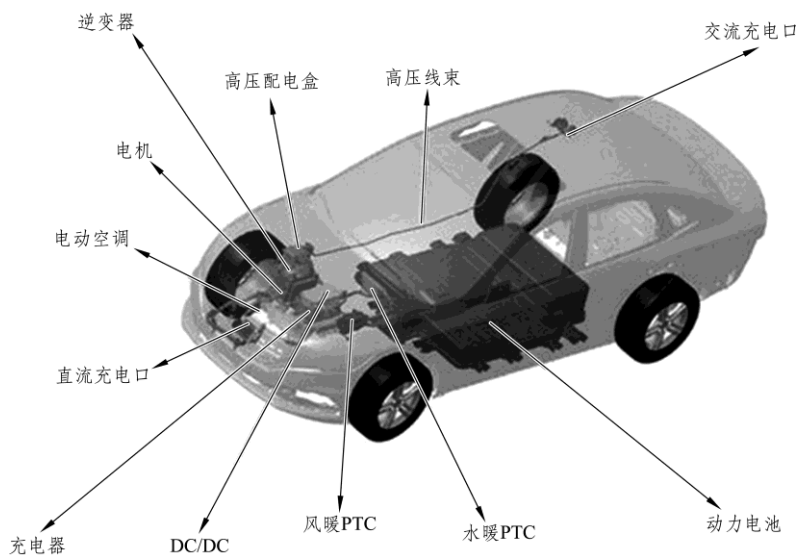
图 1-17 纯电动汽车高压系统
