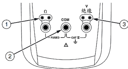
图 1-13 输入端子
