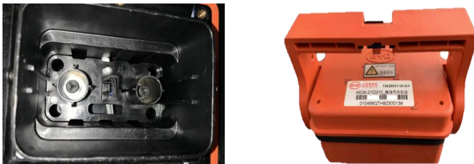
图 1-23 维修开关
